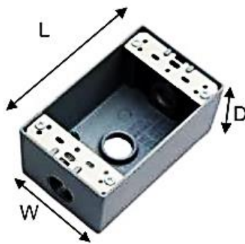
3 salidas/agujeros
